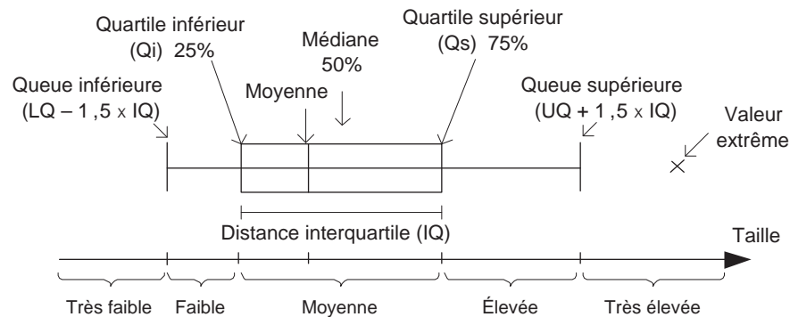
FIG. 3.6 – Le boxplot.
