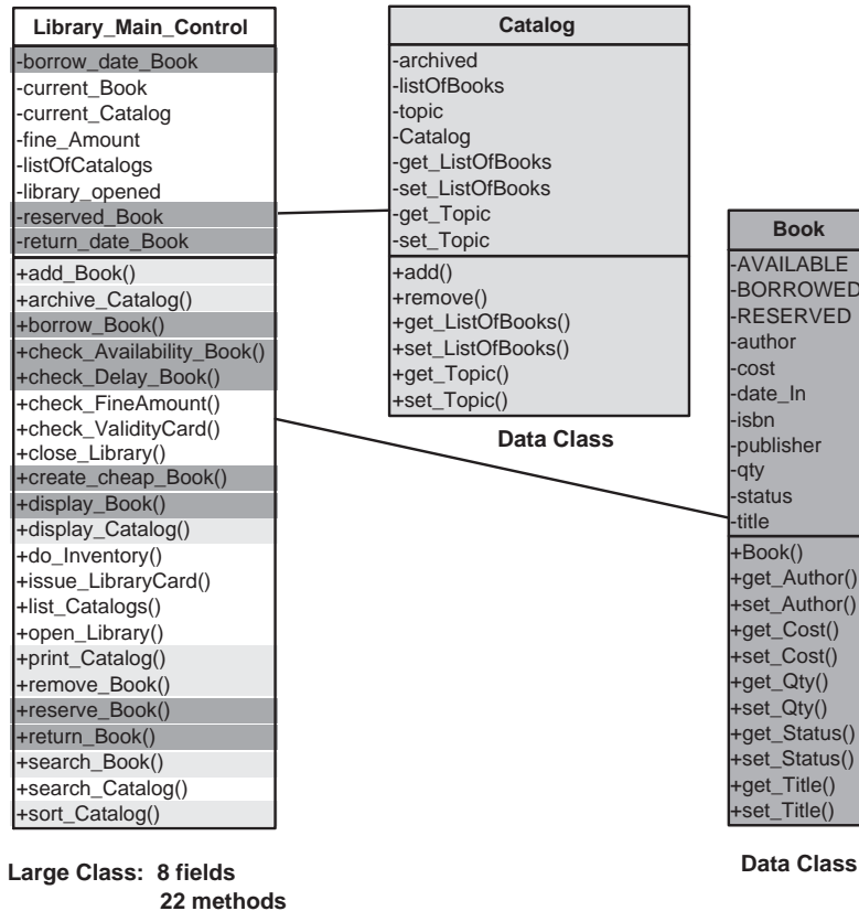
FIG. 4.4 – Diagramme de classes du Blob lié à la gestion d’une bibliothèque (les attributs et méthodes en gris foncé et en gris clair de la classe Library_Main_Control sont des membres de classe qui sont associés respectivement aux classes de données Book et Catalog ).
